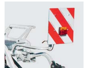
Beleuchtung Warntafeln
